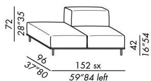
elemento penisola / penisula unit 155
