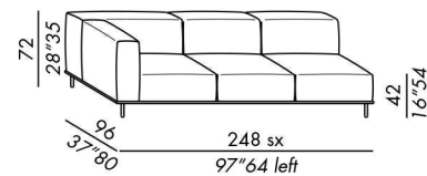
elemento angolo / corner unit 250
