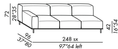
terminale / end unit 250
