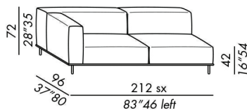
elemento angolo / corner unit 215
