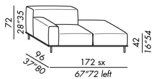
terminale penisola / penisula end unit 175
